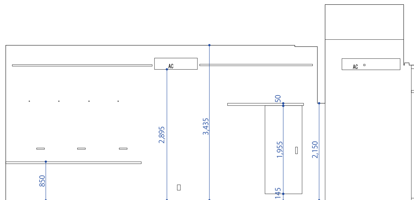
■ B1断面図
