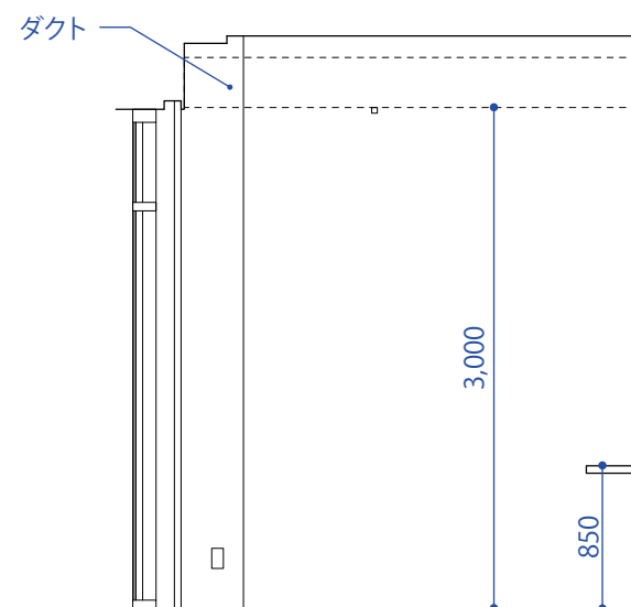
■ B2断面図
