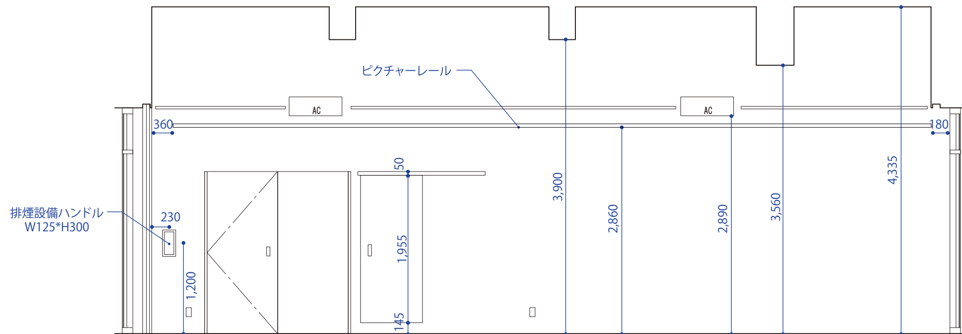
■ A1断面図
