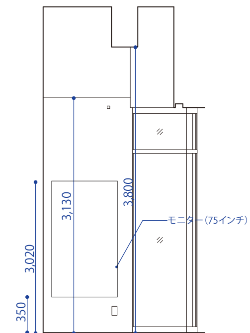
■ A2断面図
