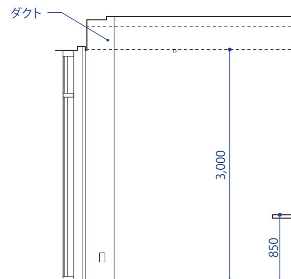
■ B2断面図
