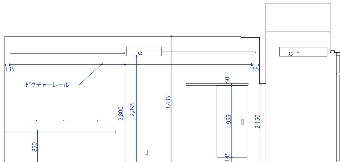
■ B1断面図
